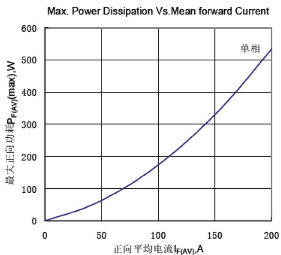
Fig.3 最大正向功耗与平均电流关系曲线
